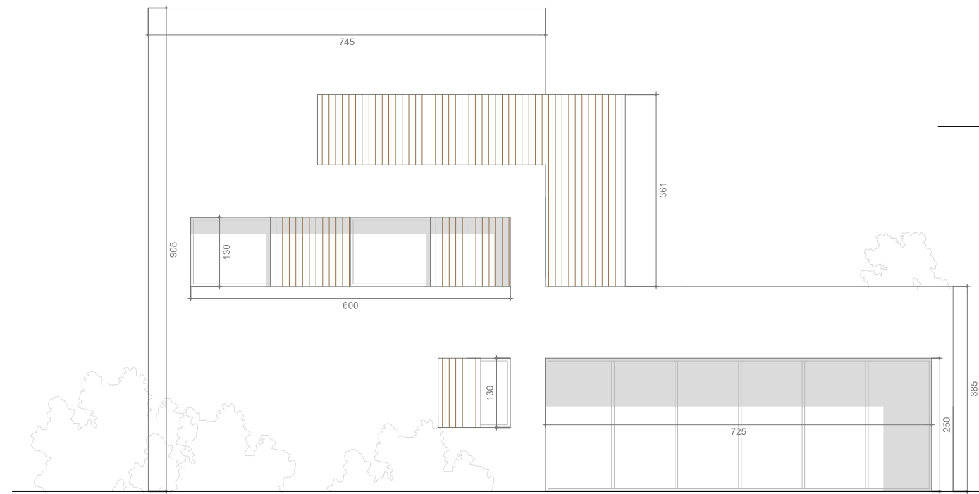
PROSPETTO NORD
