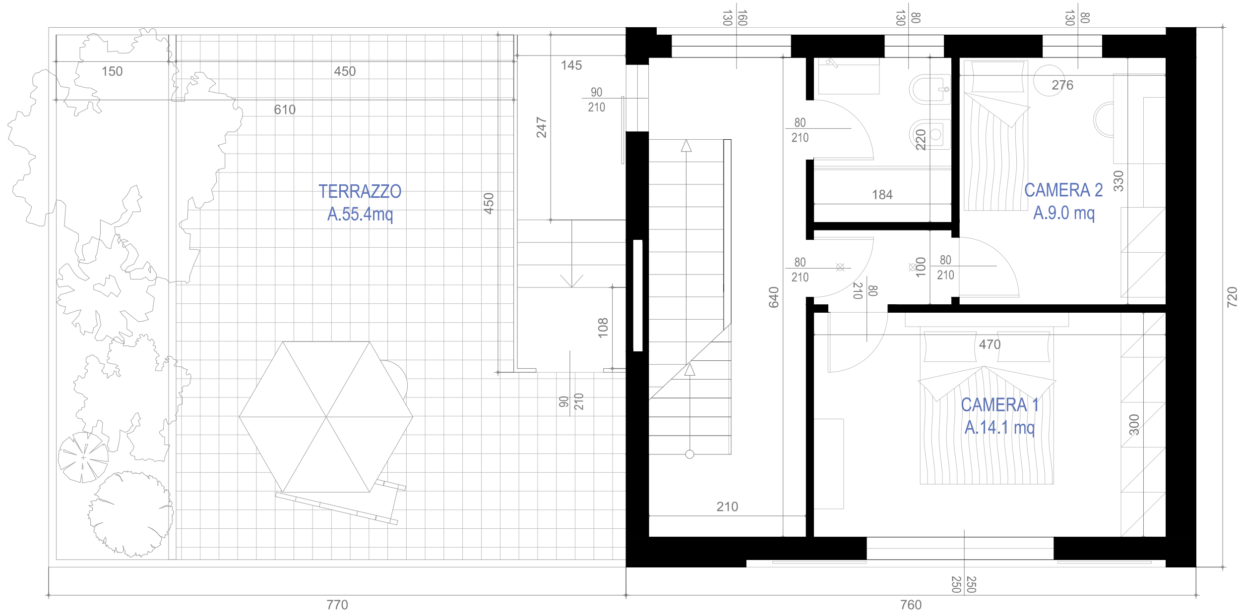
PIANO PRIMO
